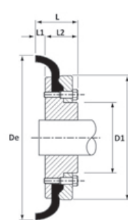
Voorgeboorde flens type B
