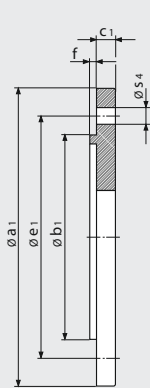
Flange B5 (1)
